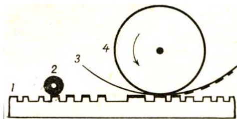
Рис. 4. Схема высокой печати:
